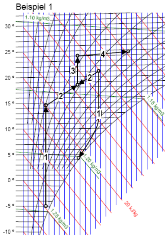
Rekuperativ-WRG, Mischung Nachwärmung, Dampfbefeuchtung
