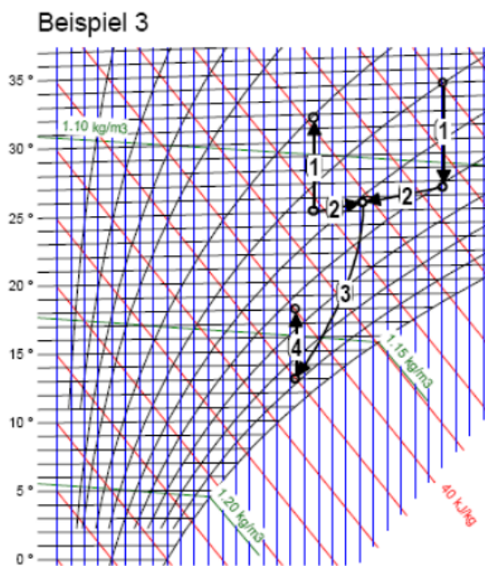
Rekuperativ-WRG, Mischung Kühlung, Nachwärmung
