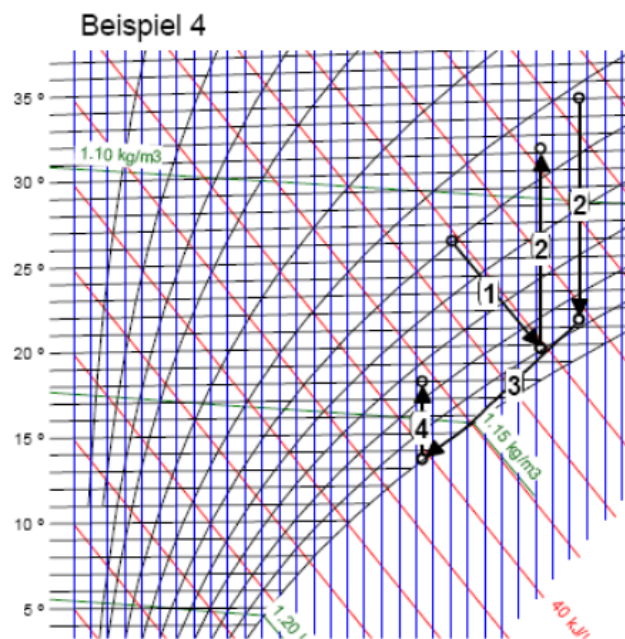
adiabate Befeuchtung, Rekuperativ-WRG Nachkühlung, Nachwärmung
